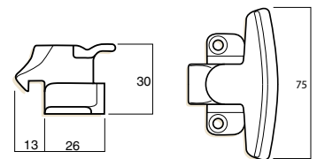
Non lockable
